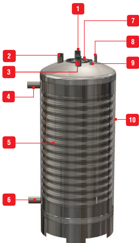
Водонагреватель показан без теплоизоляции
