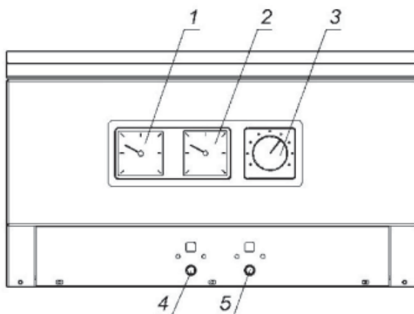
Рисунок 4. Внешний вид панели управления котла котла ALFA COMFORT v15 .
